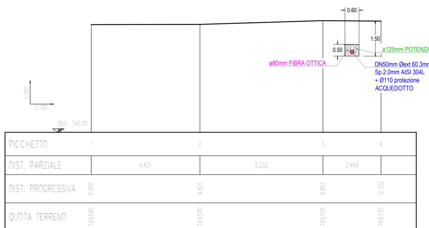
SEZ. 1-1
