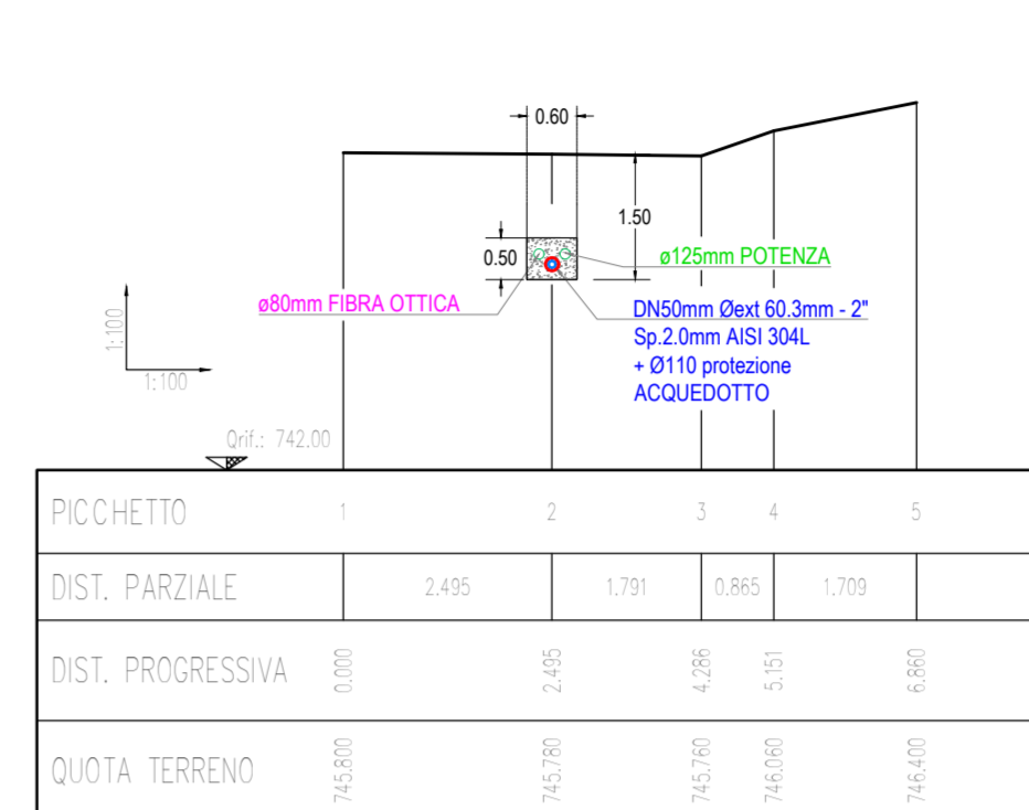
SEZ. 3-3
