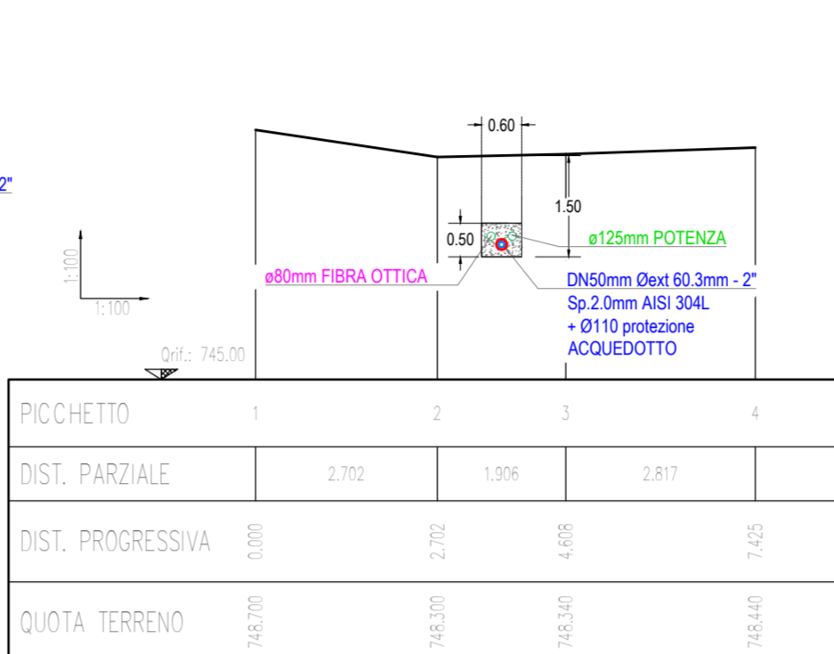
SEZ. 2-2
