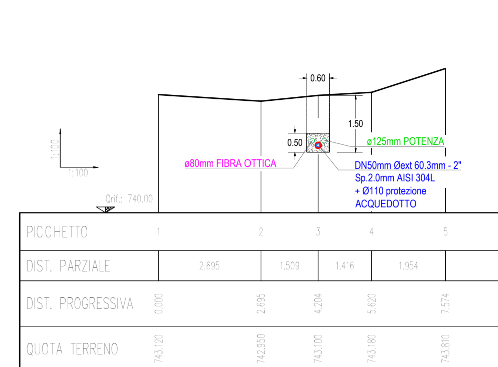
SEZ. 4-4
